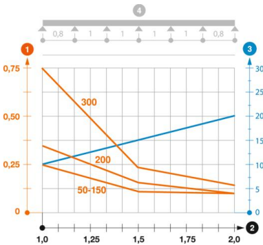
Diagrama de cargas do caminho de cabos GR-Magic do tipo GRM 35
